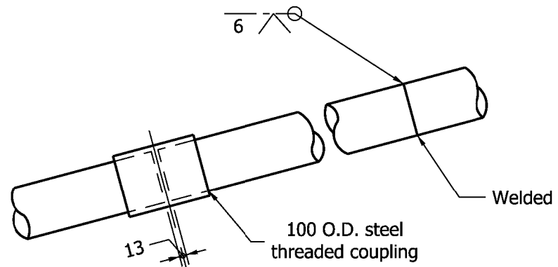
OPTIONAL COUPLING
